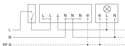
Diagrama electrónico lámpara sin conductor neutro
